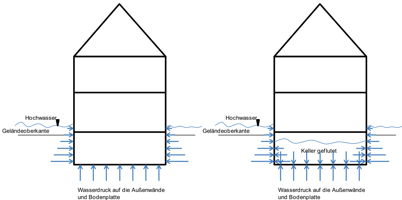
Abb. 13: Belastung durch den Wasserdruck bei einem leeren und einem gefluteten Keller
