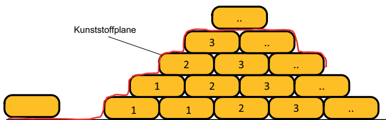
Abb. 12: Sandsackdamm mit eingebauter Plane
